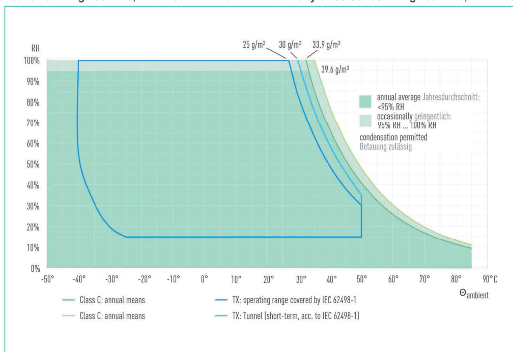
Klimaklasse Baureihe MKPg 265 / 275, MKP 266.1-7 / 276.1-7
