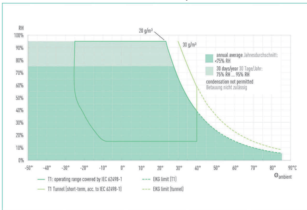
Klimaklasse Baureihe MKP 276.0
